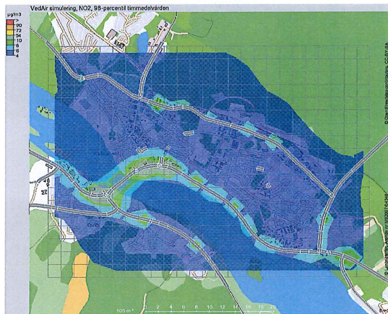
Figur 5: 98-percentil av timmedelhalt av NO 2 för Kalix tätort.
