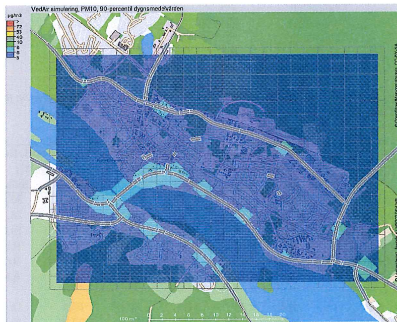
Figur 2: 90-percentil av dygnsmedelhalt av PM10 för Kalix tätort.
