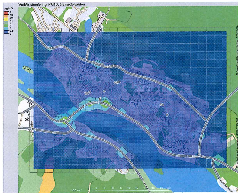
Figur 1: Årsmedelhalt av PM10 för Kalix tätort.
