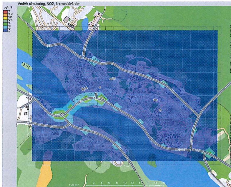
Figur 3: Årsmedelhalt av NO 2 för Kalix tätort.
